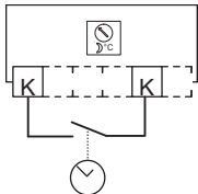
Рис.4 Подключение таймера ночного режима
